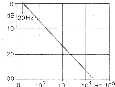
Pink Noise Option SUF 2-Z3
