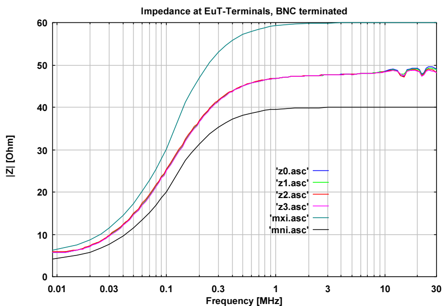
Abb. 5 Impedanz an den Prüflingsklemmen, BNC mit 50 \Omega Abschluss Impedance of connector for DuT, BNC terminated with 50 \Omega
