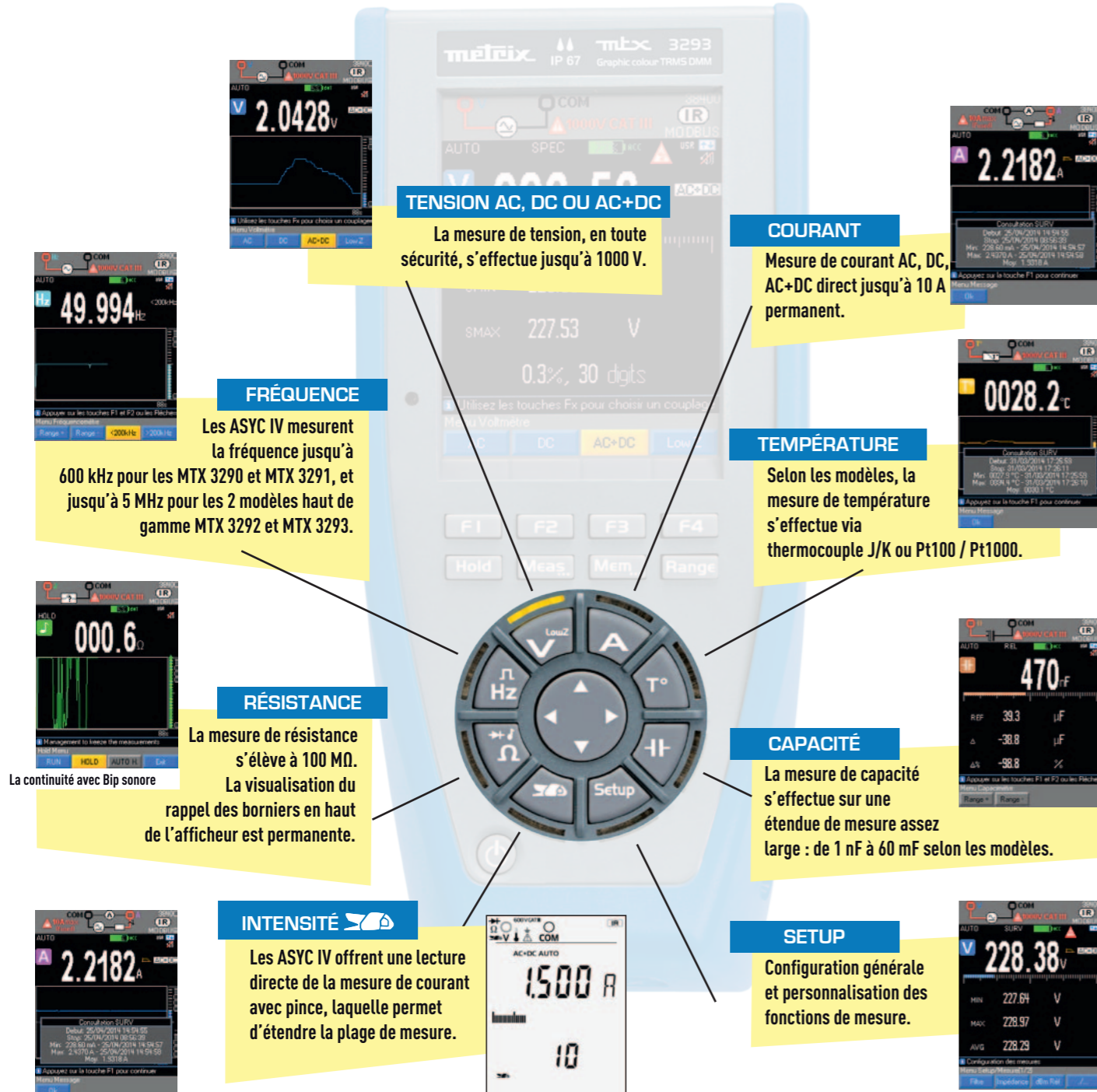
Rapport paramétrable mV/A ou A/A sur MTX 3292/3293
