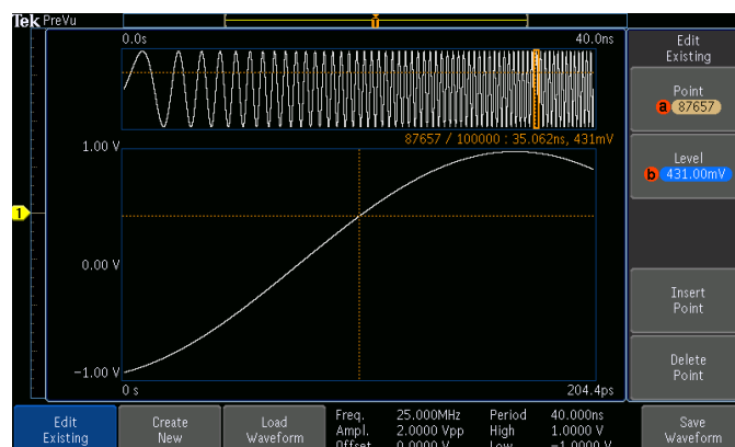
Éditeur de signaux arbitraires point par point.
