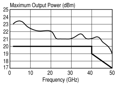
83050A Amplifier
