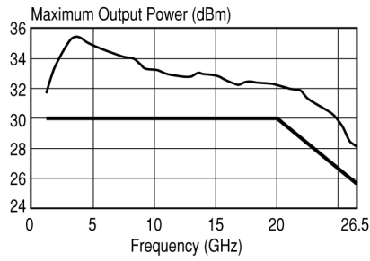
83020A Amplifier
